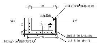
施工斷面圖 S=1/50
