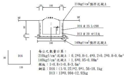
施工斷面圖(二) S=1/50 Unit: cm
