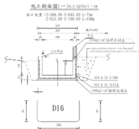
施工斷面圖(數量計算)每m
