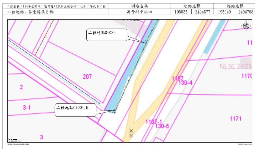
工程位置圖
